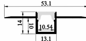
SJ-ALP5213-FLEX
