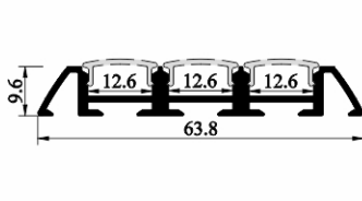
SJ-ALP6009B
