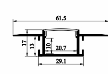
SJ-ALP6117
