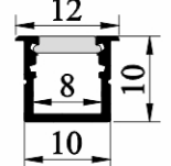
SJ-ALP1210
