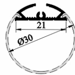
SJ-ALPO3030
