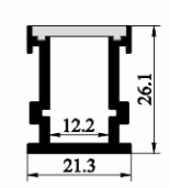
SJ-ALP2621
