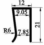
SJ-ALP1221
