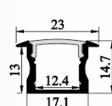
SJ-ALP2515B
