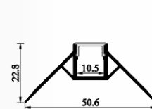
SJ-ALP4822
