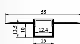
SJ-ALP5515
