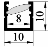
SJ-ALP1010-30D
