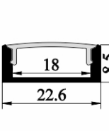
SJ-ALP2208
