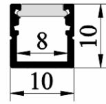
SJ-ALP1010
