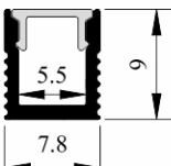
SJ-ALP0809
