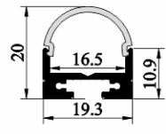
SJ-ALP2119
