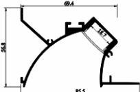
SJ-ALP8570
