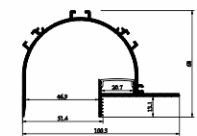
SJ-ALP10168
