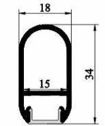
SJ-ALP1834
