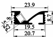
SJ-ALP2409
