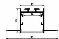
SJ-ALP3535-R8
