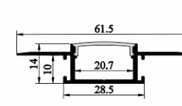
SJ-ALP6114
