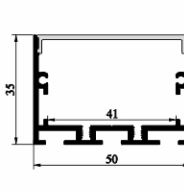
SJ-ALP5035
