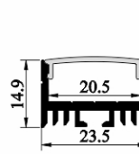
SJ-ALP2415
