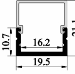
SJ-ALP2016B
