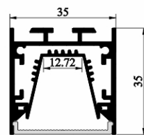
SJ-ALP3535-R6
