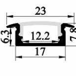
SJ-ALP2508
