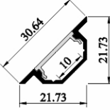
SJ-ALP2222
