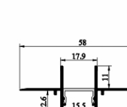
SJ-ALP5825
