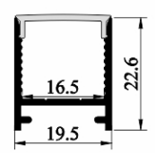
SJ-ALP2023
