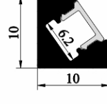
SJ-ALP1010C
