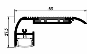
SJ-ALP6528
