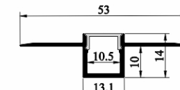
SJ-ALP5213
