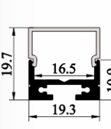
SJ-ALP2119B
