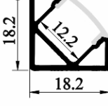
SJ-ALP1919F
