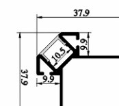
SJ-ALP3927
