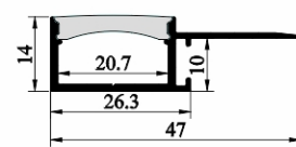
SJ-ALP4714-FLEX
