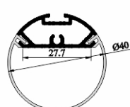
SJ-ALPO4040
