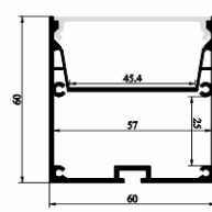
SJ-ALP6060-R1
