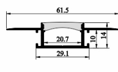
SJ-ALP6114-FLEX
