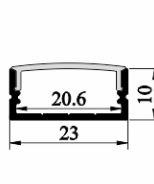
SJ-ALP2310
