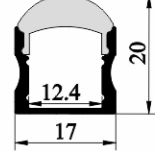
SJ-ALP1715C
