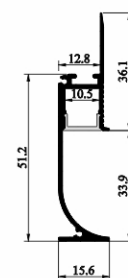
SJ-ALP7016
