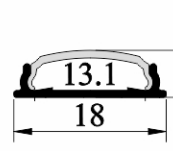
SJ-ALP1806
