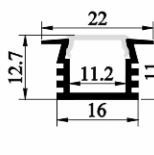
SJ-ALP2212
