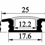
SJ-ALP2507
