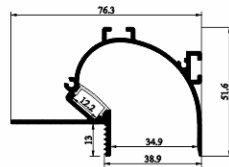
SJ-ALP7752
