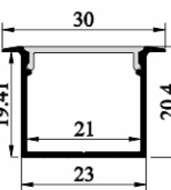
SJ-ALP3020
