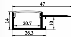
SJ-ALP4714
