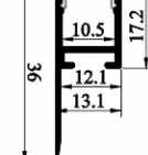
SJ-ALP3613
