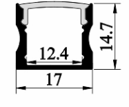
SJ-ALP1715B
