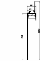
SJ-ALP18119
