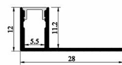
SJ-ALP2812
