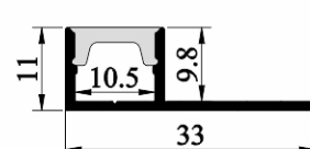
SJ-ALP3311-FLEX
