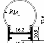
SJ-ALP2033
