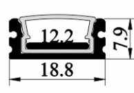
SJ-WALP1808
