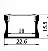
SJ-ALP2216
