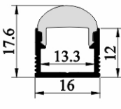
SJ-ALP1612H
