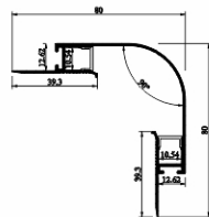
SJ-ALP8080C
