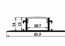
SJ-ALP6114B
