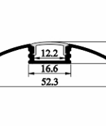
SJ-ALP5208
