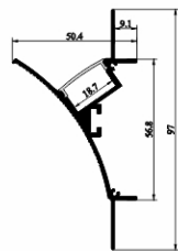
SJ-ALP9635R
