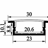
SJ-ALP2910
