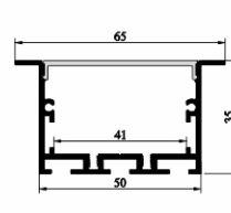
SJ-ALP6535
