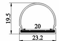
SJ-WALP2319
