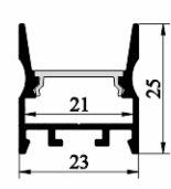
SJ-ALP2325B
