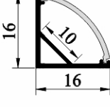
SJ-ALP1616
