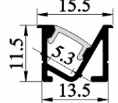
SJ-ALP1511
