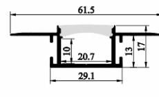
SJ-ALP6117-FLEX
