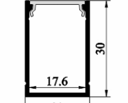
SJ-ALP2030
